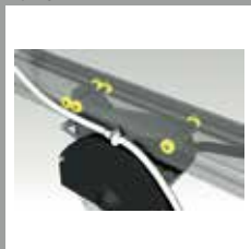
Tête de coupe montée sur 6 roulements (dont 2 ajustables) = précision de coupe absolue
