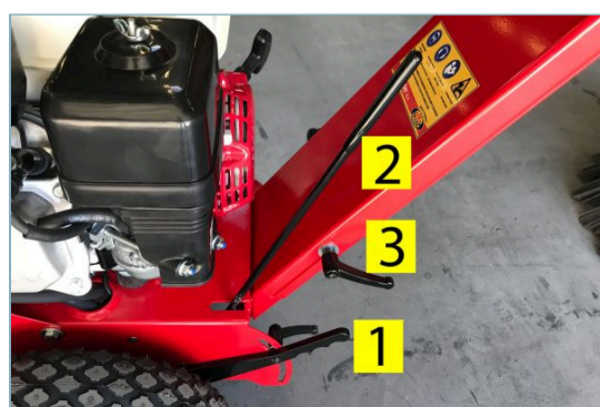
Roues/poignée réglables - Brosse rotative G/D
