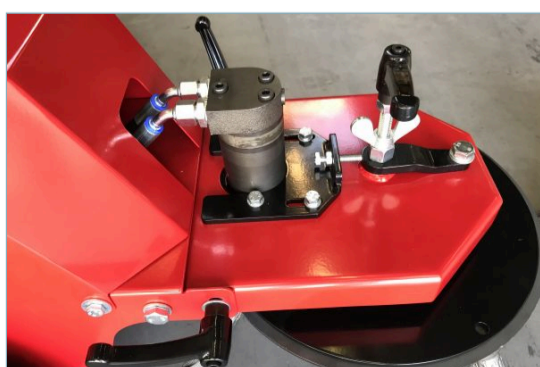
Entraînement hydraulique de la brosse
